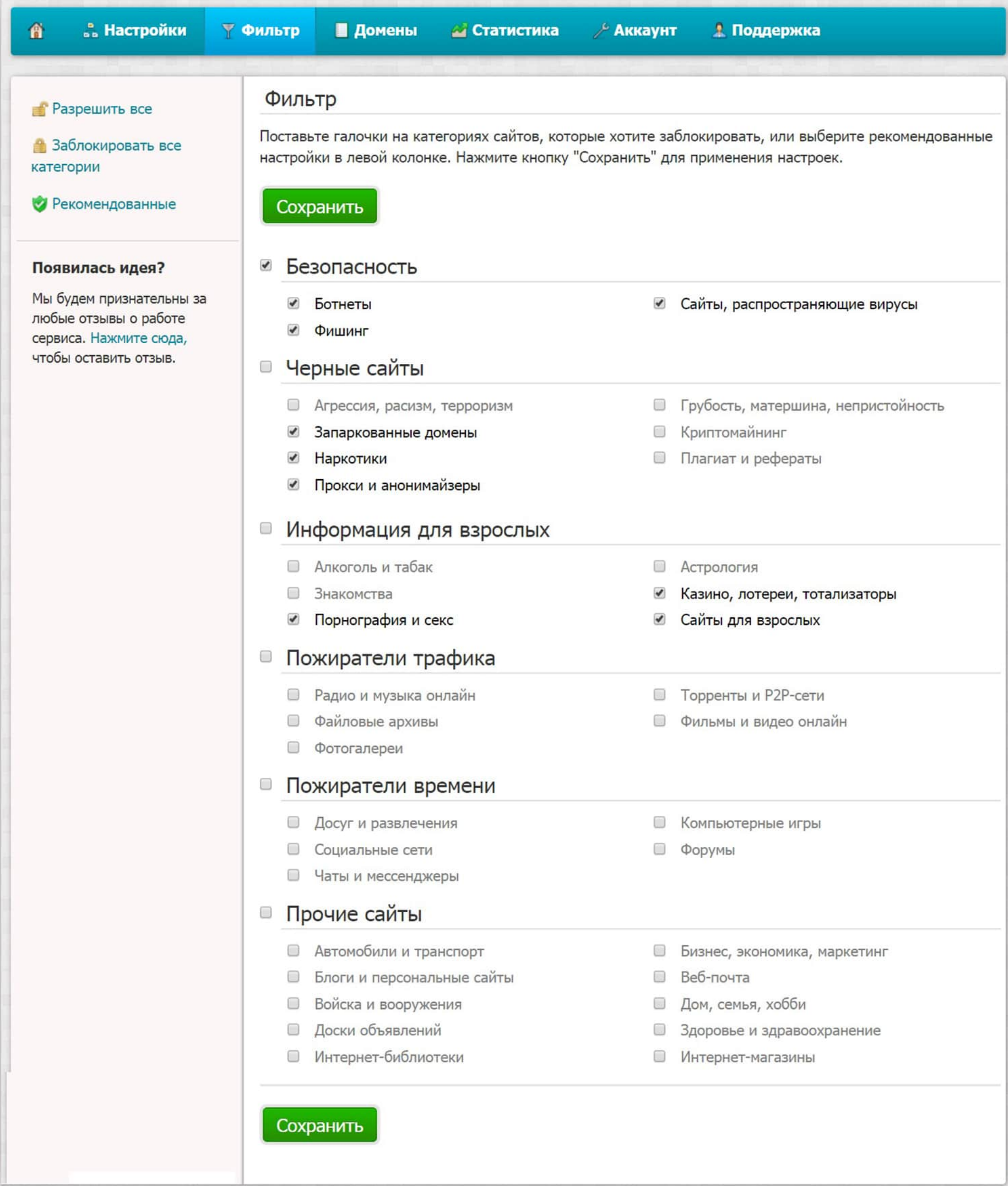
Интерфейс личного кабинета
